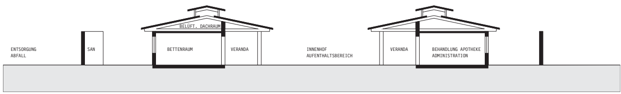
SCHNITT 1:100
