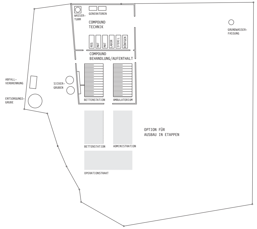
SITUATION 1:500 GESAMTPARZELLE
