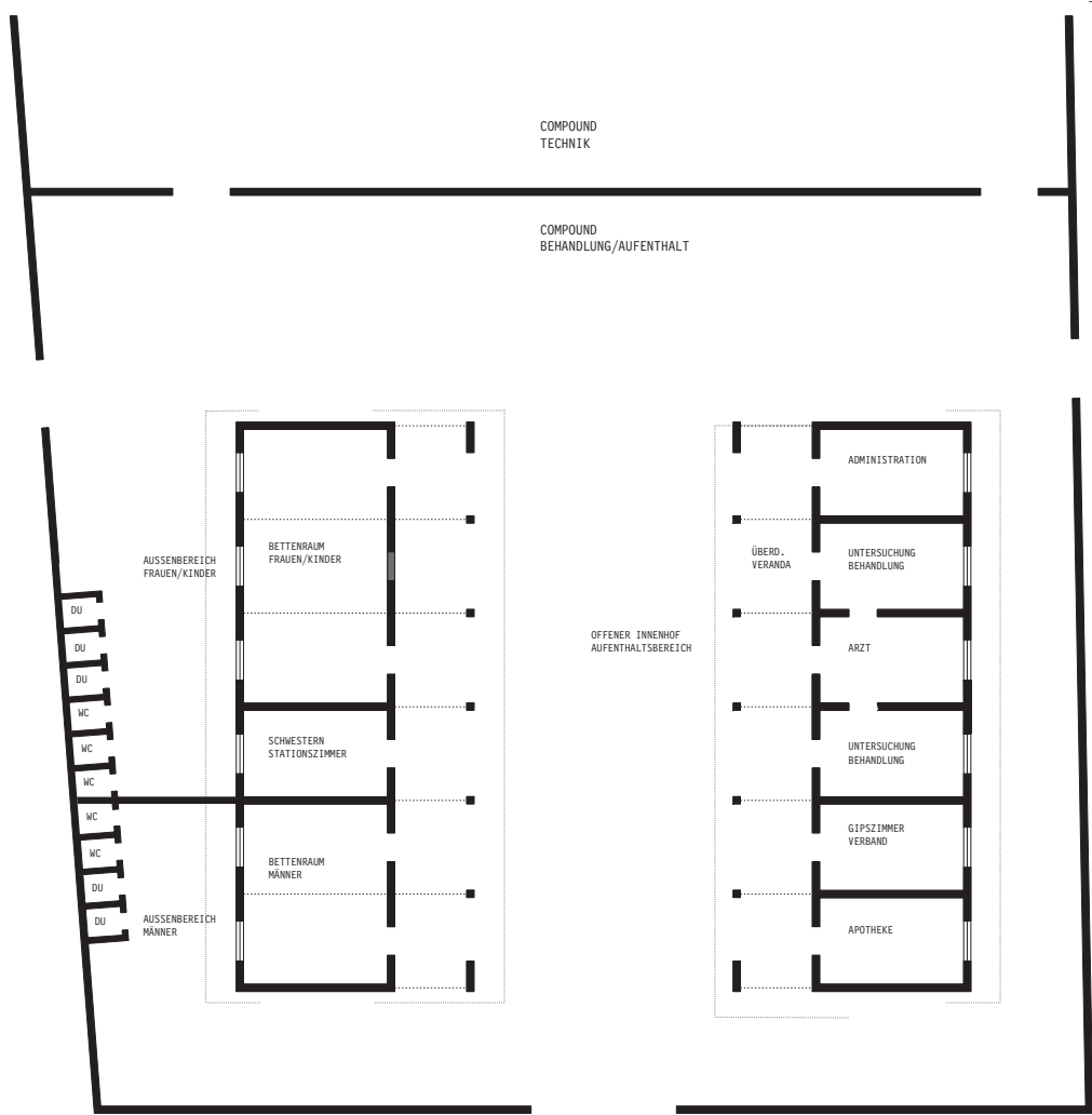
GRUNDRISS 1:100
